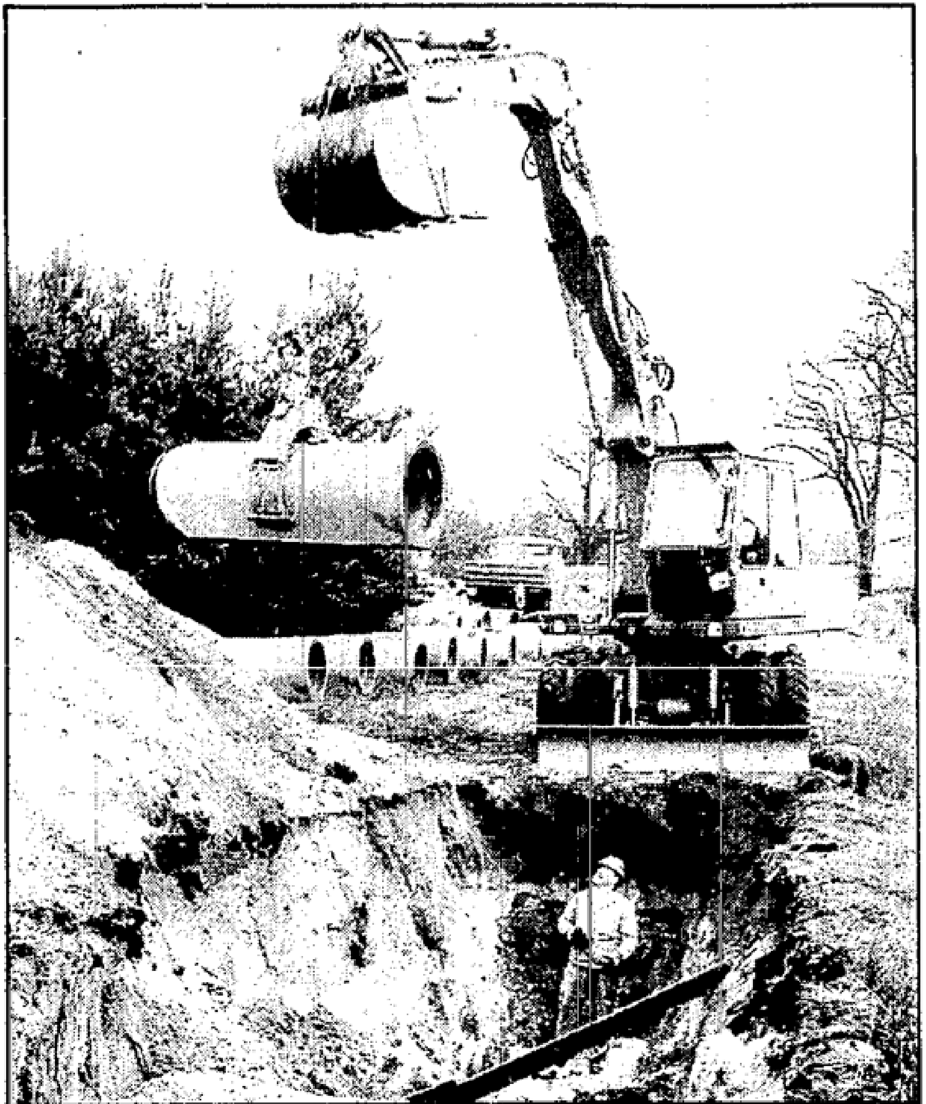
In der Radinkendorfer Straße von Beeskow wird gebuddelt. Hier wird bereits die Regenwasserleitung vom Gewerbegebiet Charlottenhof zur Spree verlegt.
