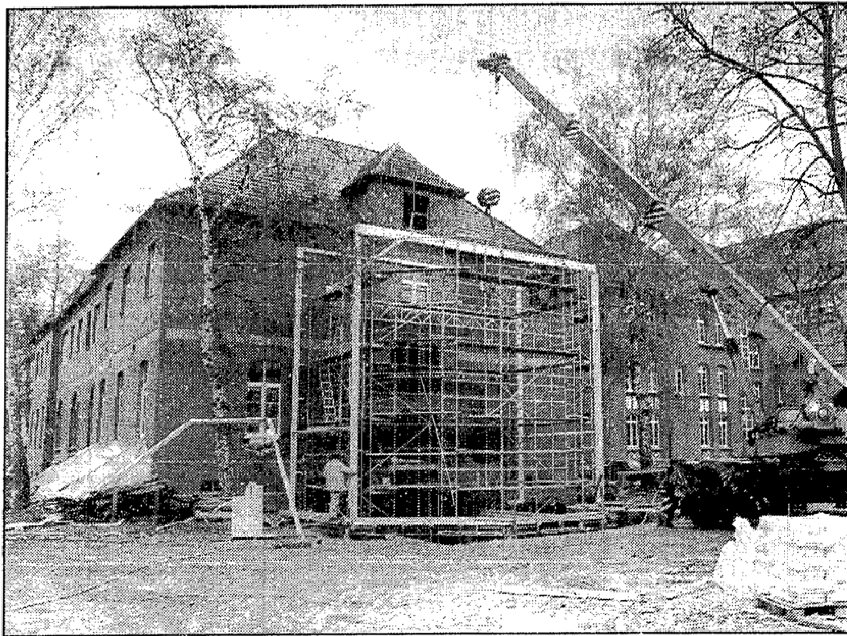
Ganz aus Glas soll der Eingang zum Nebengebäude des Gymnasiums gebaut werden. Das Stahlgerüst dafür wird bereits montiert. Hier sollen u. a. Unterrichtsräume fürs Gymnasium, eine Cafeteria im Obergeschoß und Räume für die Volkshochschule entstehen.
