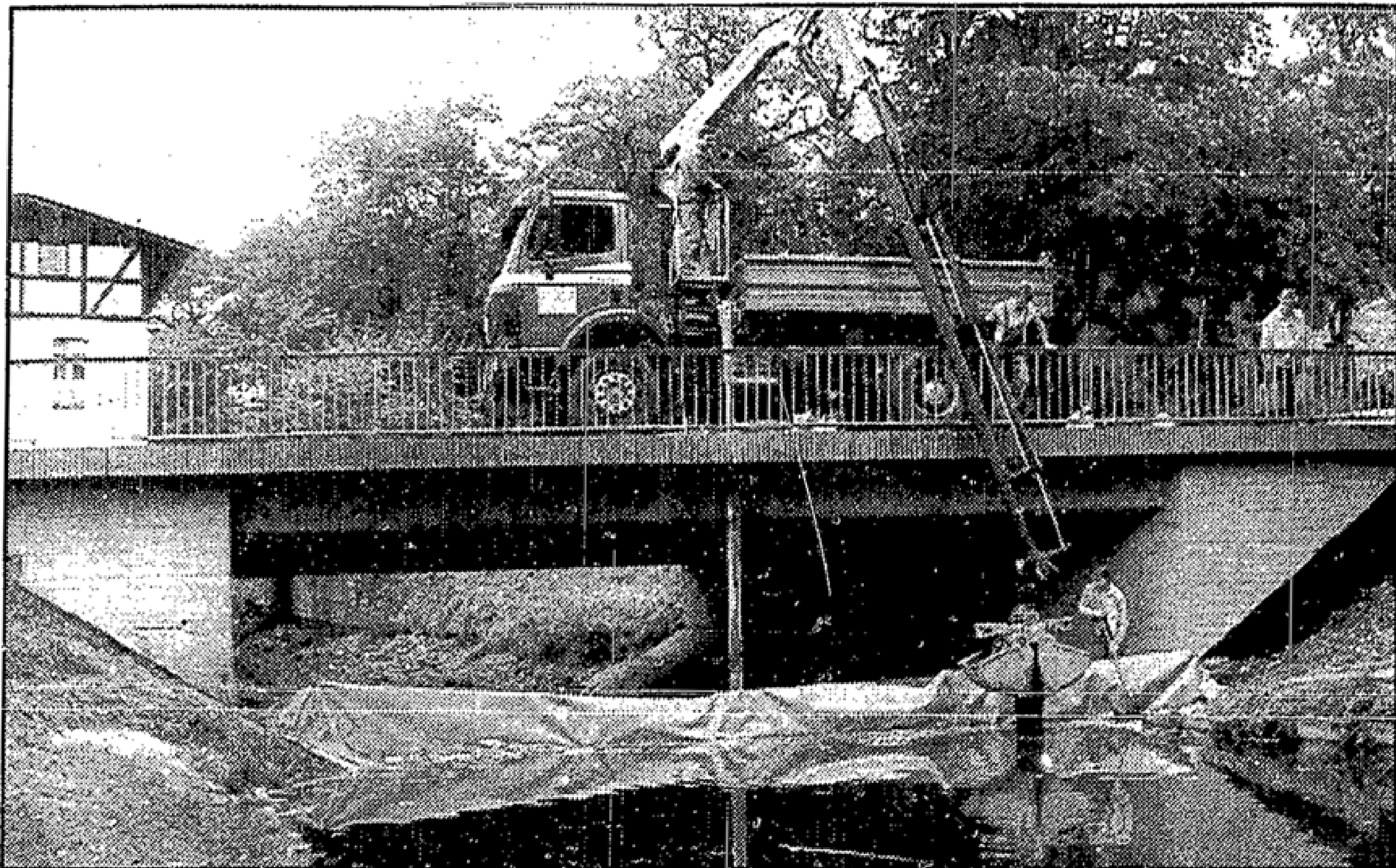
Eine neue Stützmauer aus Naturstein und Klinker auf einer Länge von 58 Meter erhält der Walkmühlen-graben in Beeskow; die alte ist seit Jahren verfallen, Erdreich drohte nachzusacken. Fotos: Karl-Heinz Arendsee
